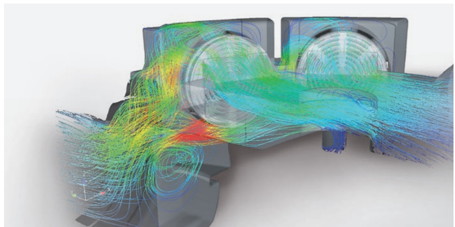
Fluid-dynamic evaluation
